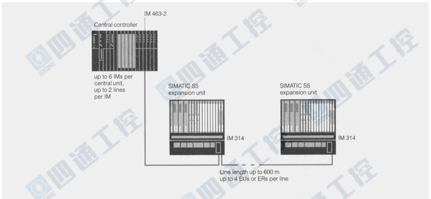
图：用 SIMATIC S5 扩展单元的扩展
