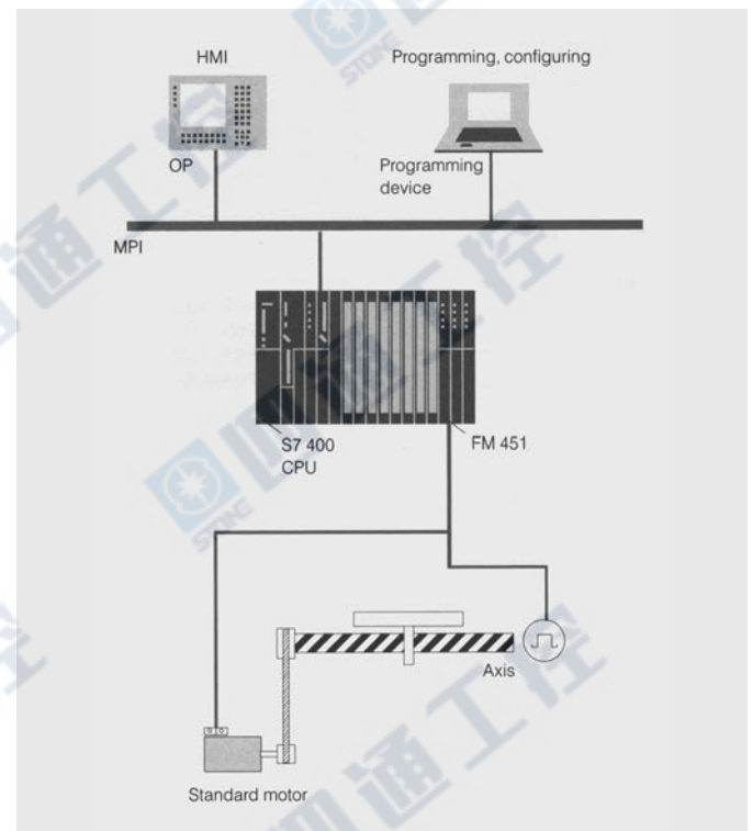
图：使用 FM451 的定位控制
