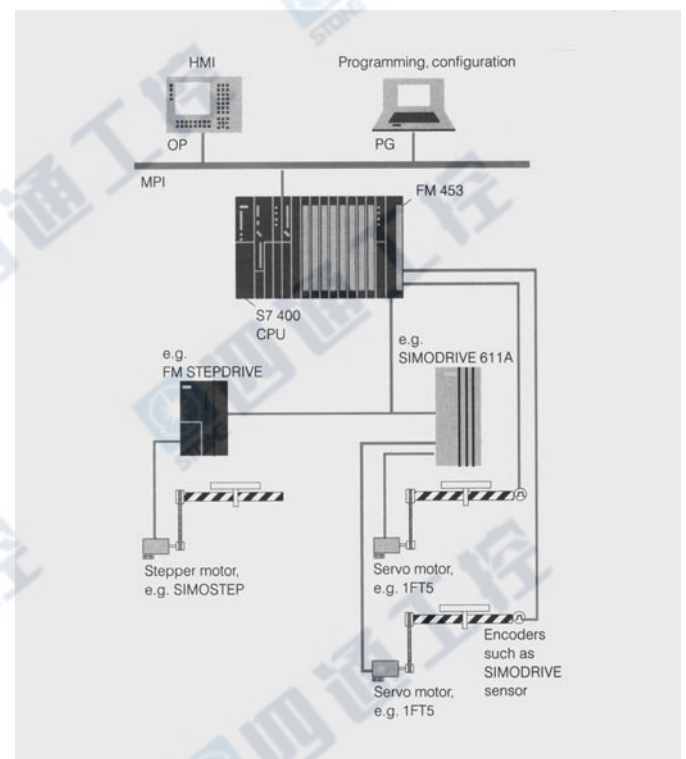
图：用 FM 453 进行定位控制的典型配置
