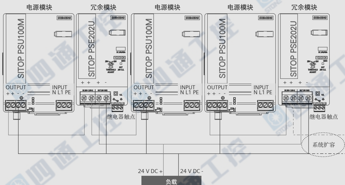
接线示意图
