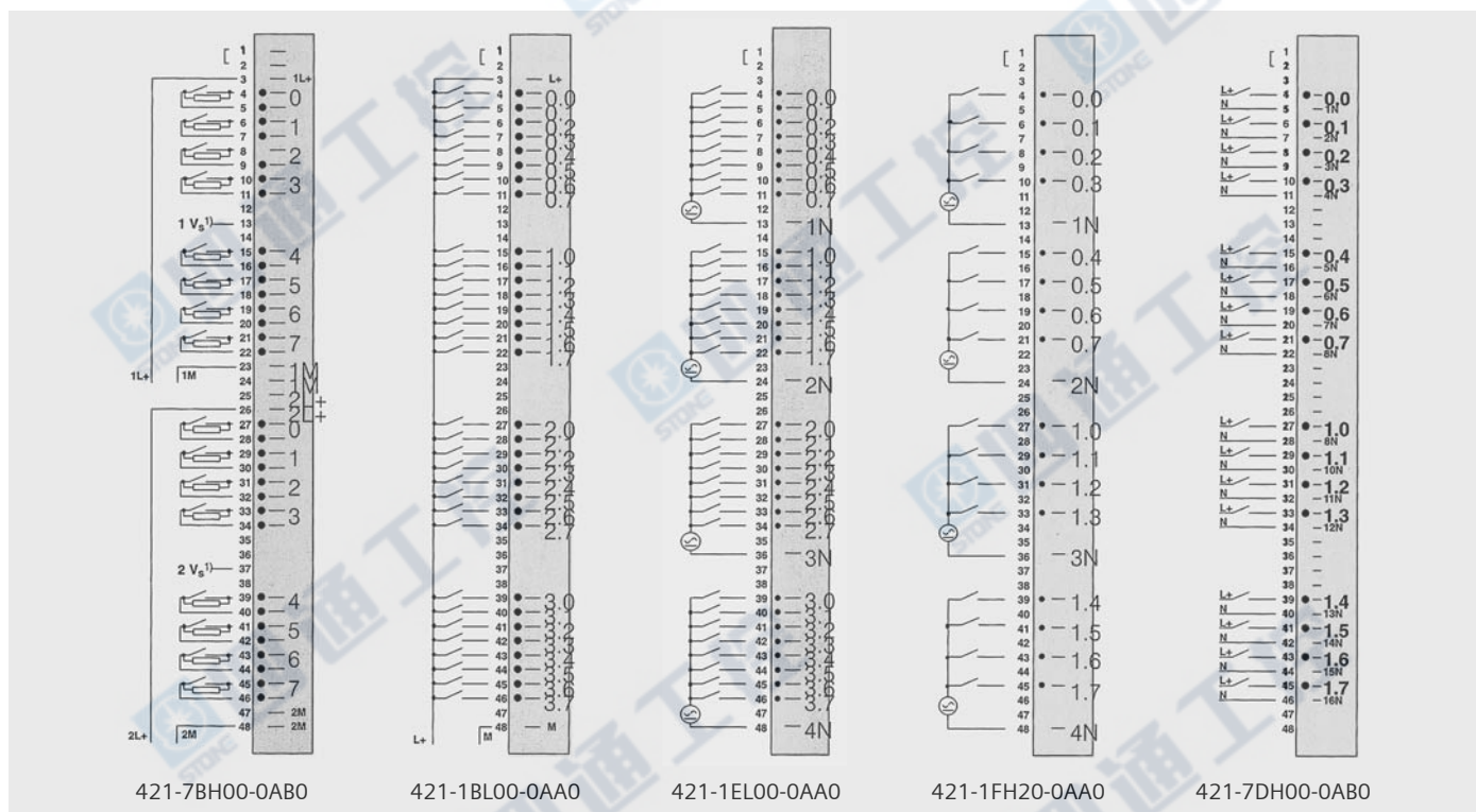
图：数字量输入模板的端子连接图
