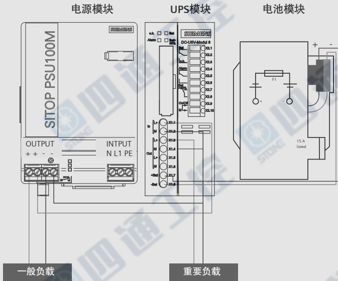
接线示意图
