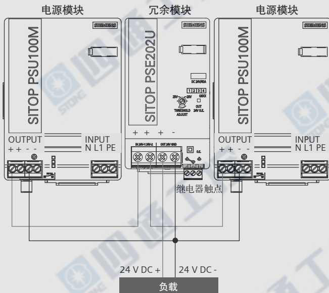
接线示意图
