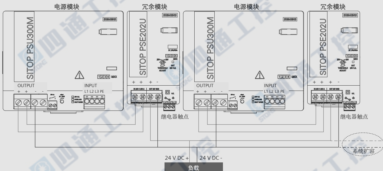
接线示意图
