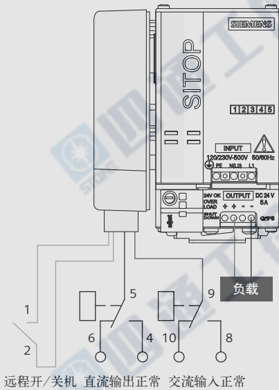
接线示意图
