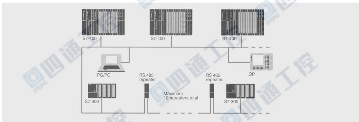
图：典型的带 MPI 接口的通讯配置
