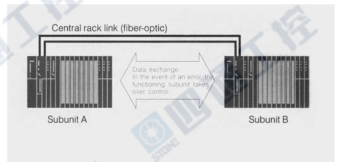
图：S7-400H 的容错通讯
