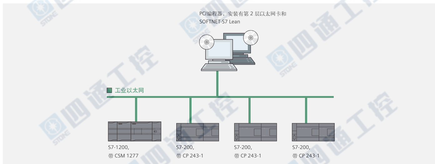
图：采用用于工业以太网的 SOFTNET-S7 Lean 和 S7-200 的系统配置
